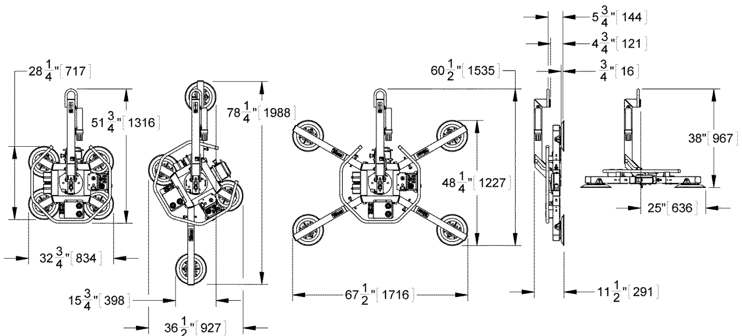
Abbildung des Hebeegerätes MRT411LDC2
