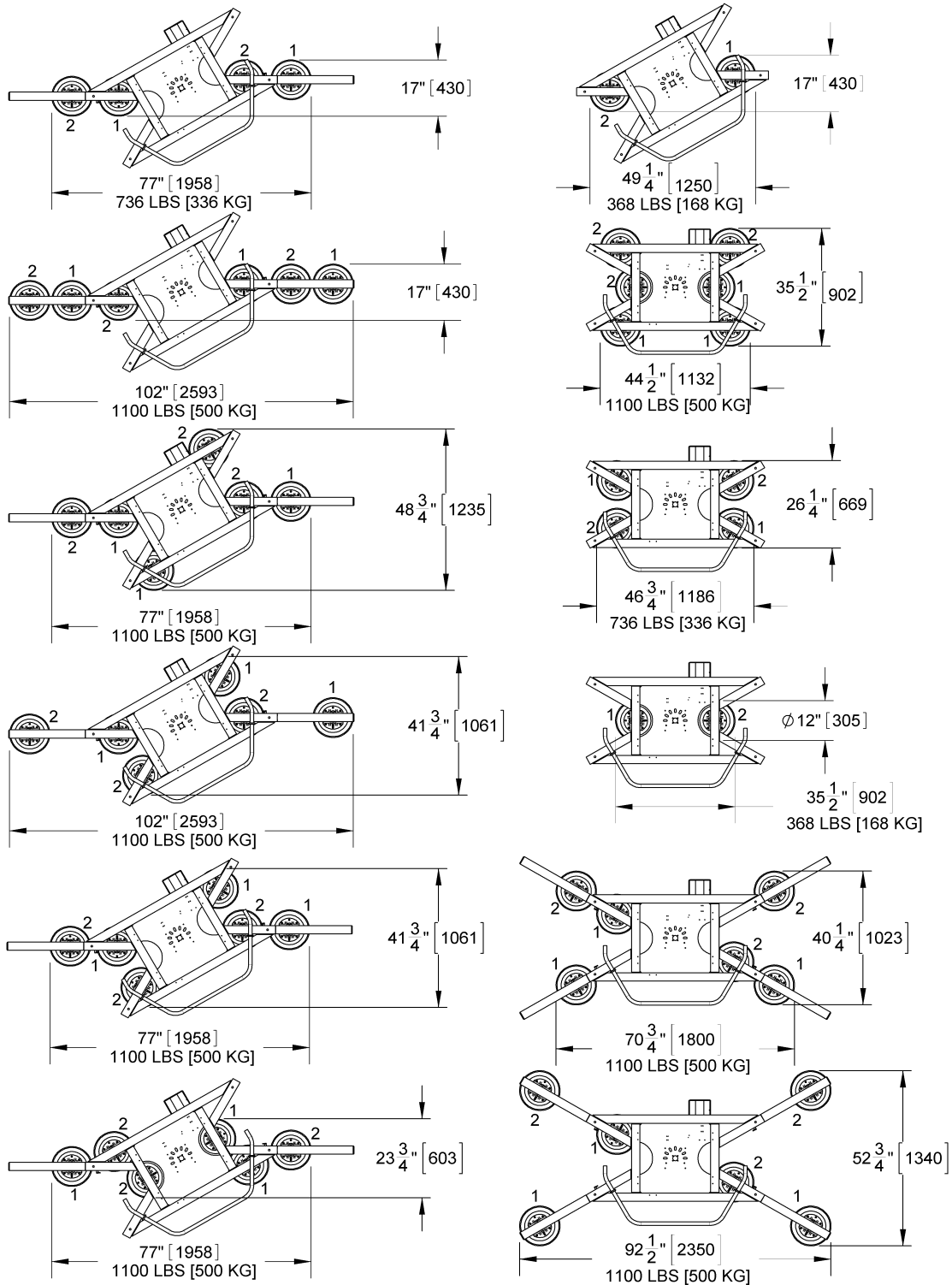
Abbildung des Saugerrahmens vom Hebegeräte MRTALP611LDC (Standard-Modell)
