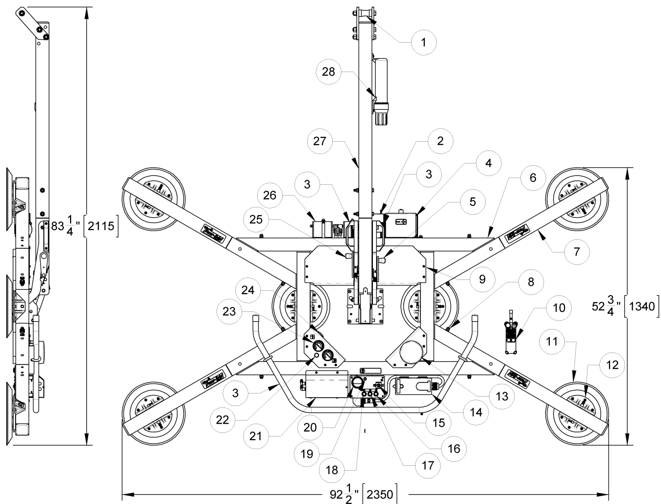
Abbildung des Hebegerätes MRTALP611LDC (Standard-Modell) mit Fernsteuerungssystem-Option.
