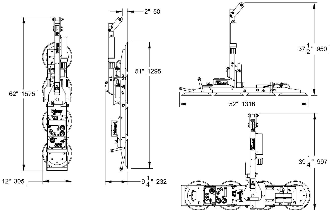
Abbildung des Hebeegerätes P11104DC2.
