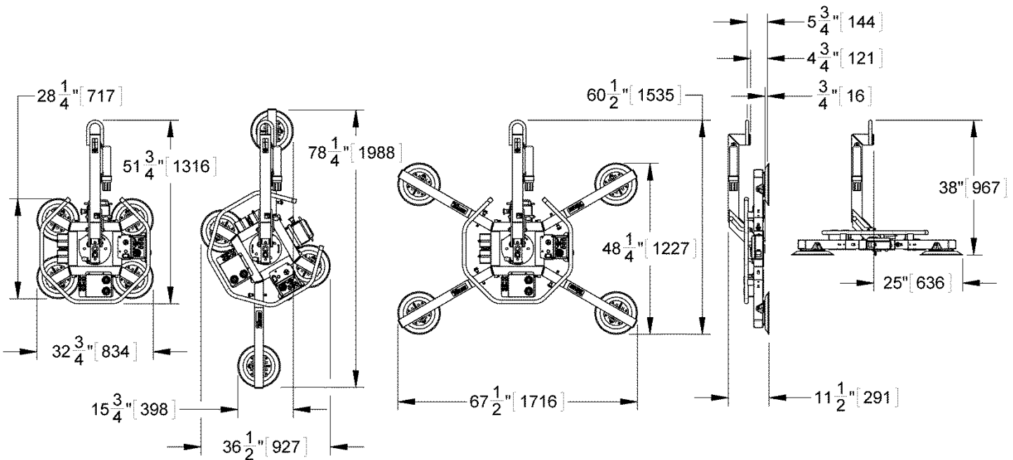
Schéma du modèle MRT411LDC2
