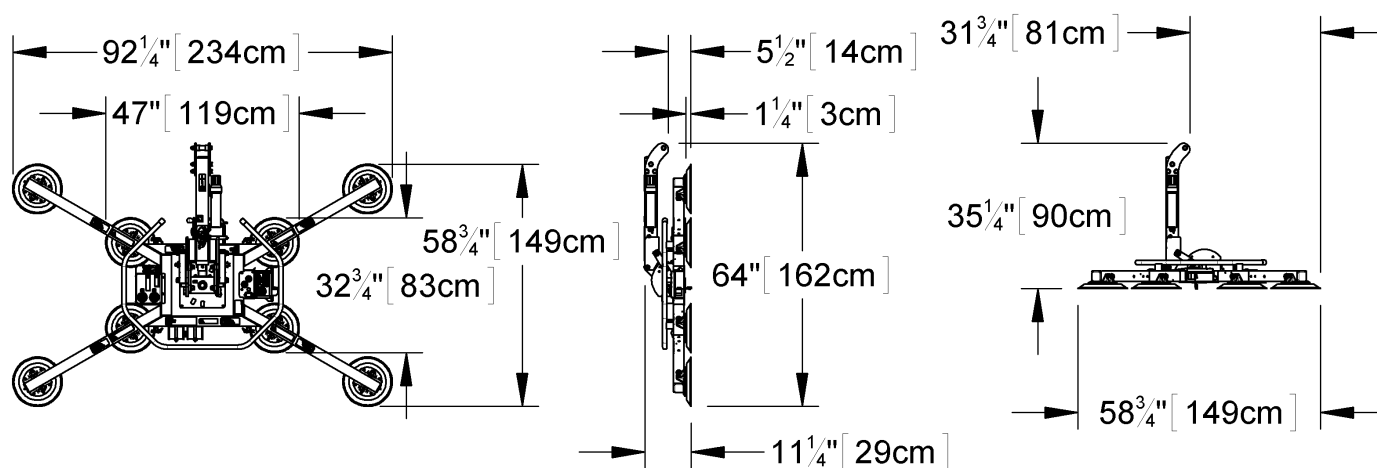
Schéma du modèle MRTA811LDC2
