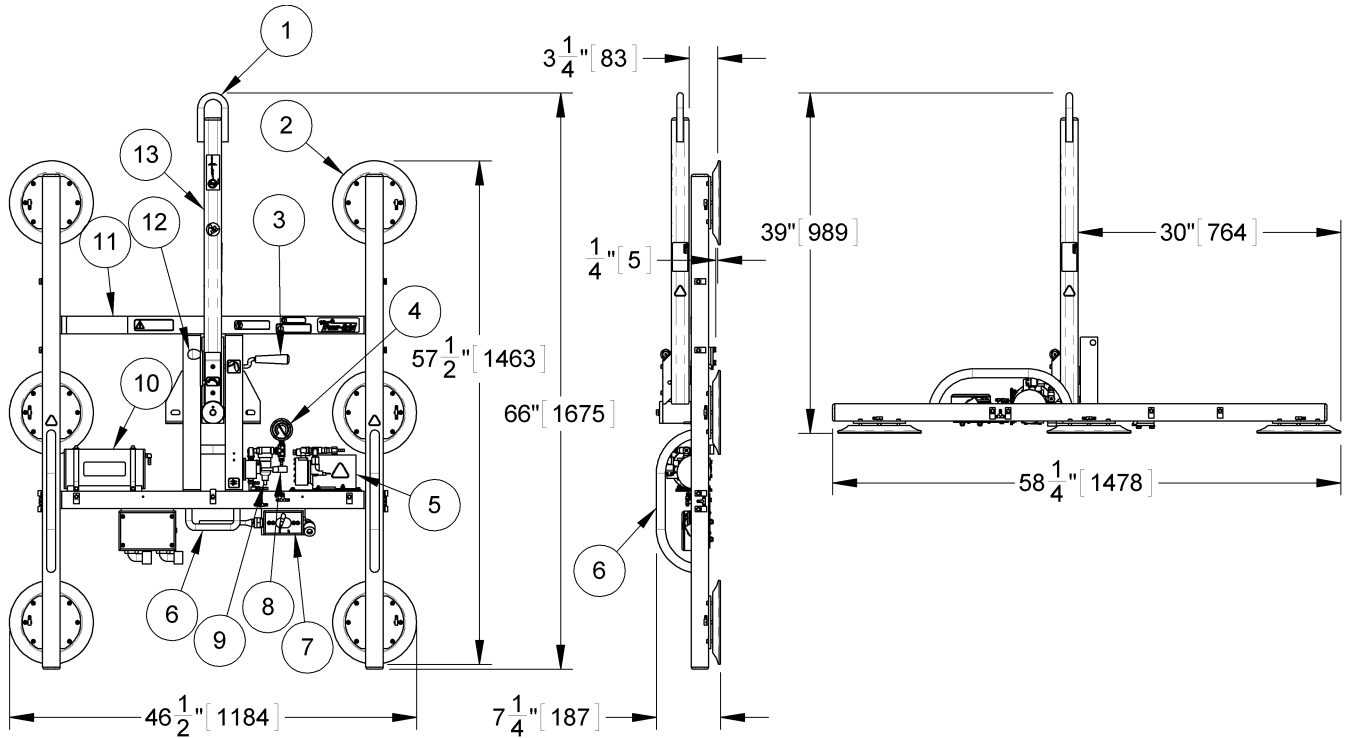
Schéma du modèle standard PFV69AC
