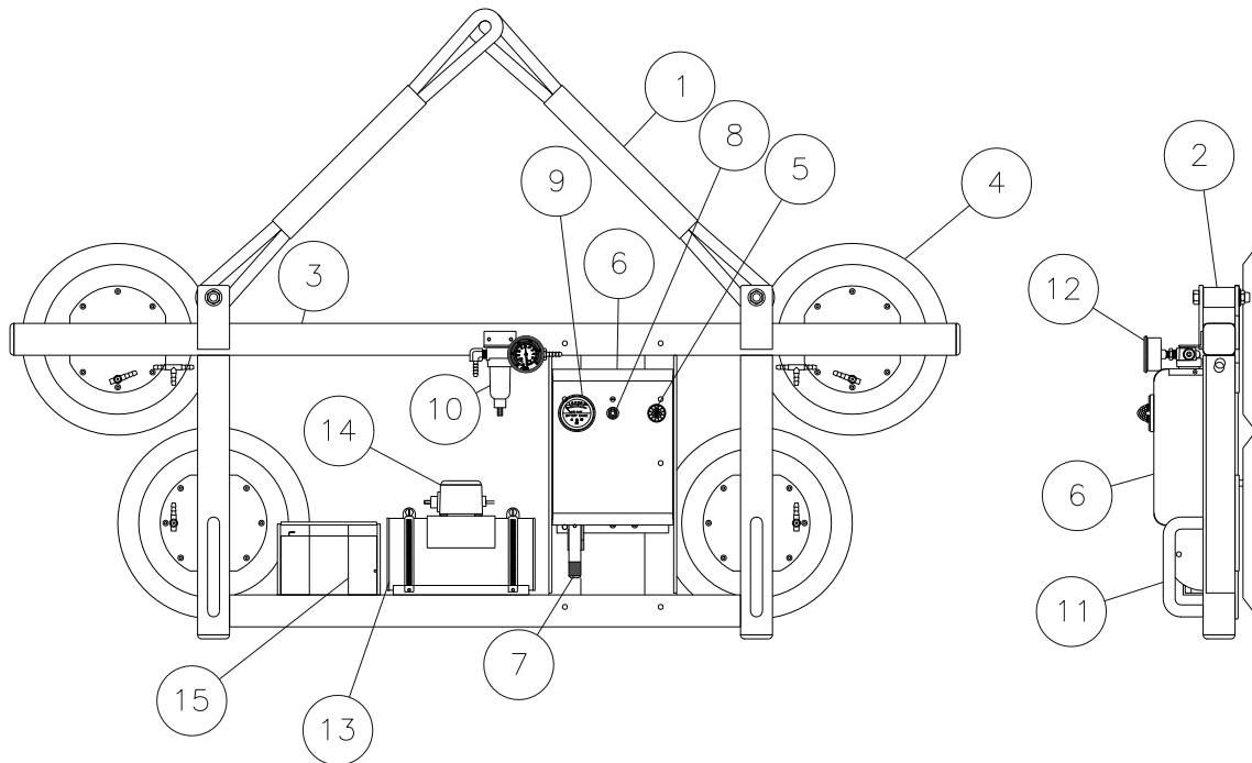
Schéma du modèle standard VL411LDC
