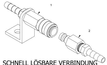
SCHNELL LÖSBARE VERBINDUNG 1 BUCHSE 2 STECKER
