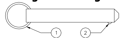
SPLINTLOSER BOLZEN 1 RING ZUM ZIEHEN 2 SPERRKUGEL
