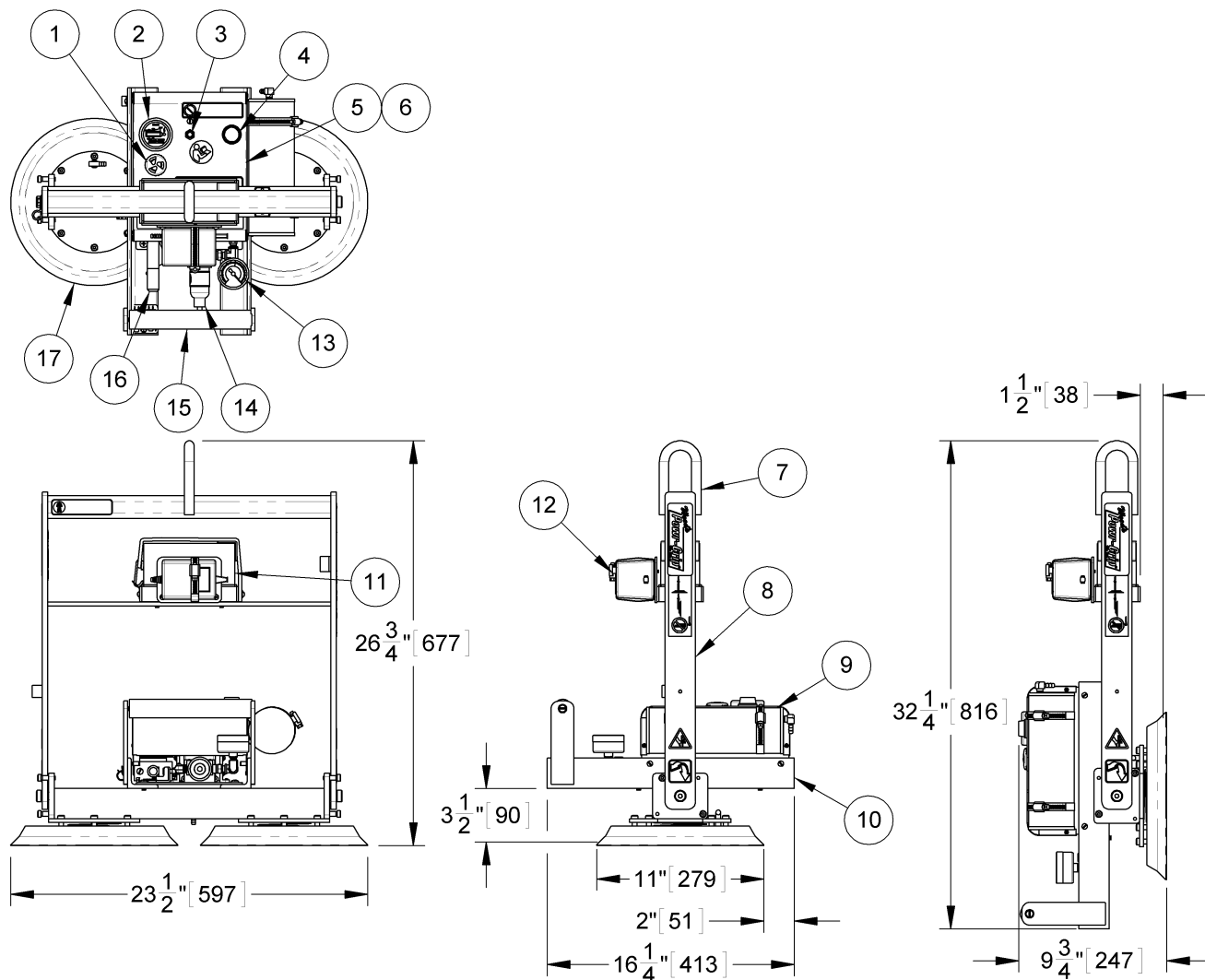
Abbildung des Hebegerätes MT2HV11DC (Standard-Modell).
