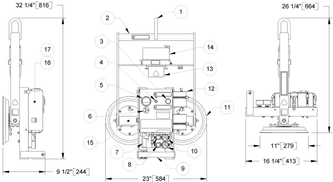
Abbildung des Hebeegerätes MT2HV11DCO (Standard-Modell) mit Doppelvakuumssystem-Option.
